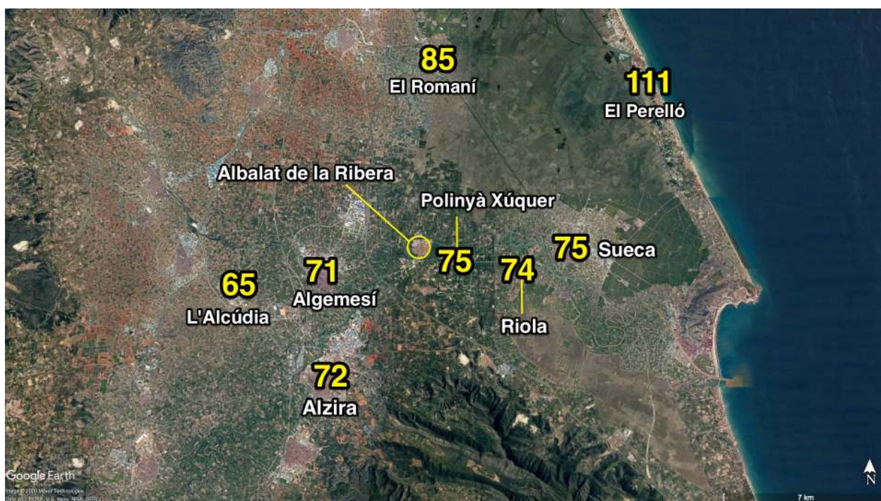
Ráfagas máximas de viento registradas en la zona de ALBALAT DE LA RIBERA y alrededores entre el 19 y el 21/01/20 (en km/h)
