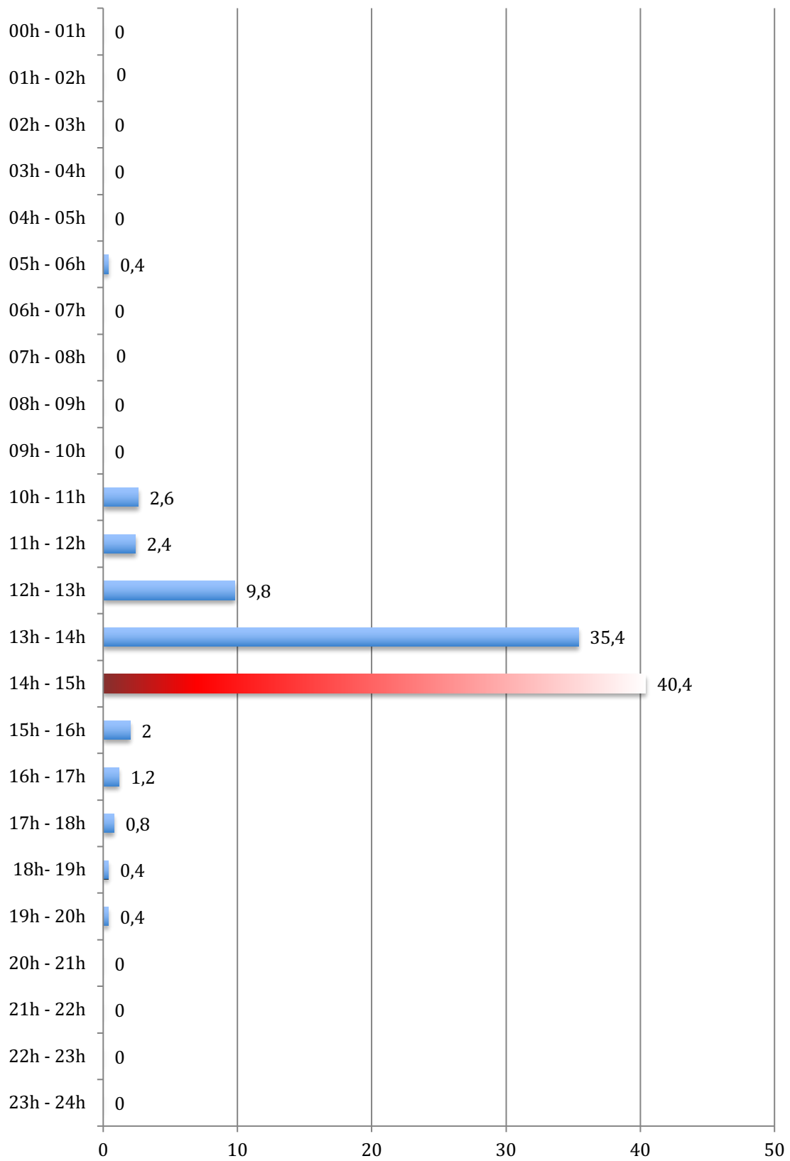
Cantidad de lluvia registrada (por horas) por la estación meteorológica el día 22/01/20 (en l/m²)
