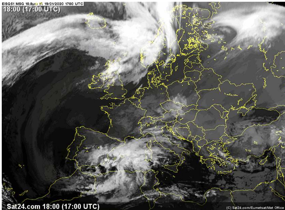
Imagen del satélite Meteosat (canal IR) a las 18:00h del 19-01-20 donde se puede apreciar la abundante nubosidad de la depresión 'Gloria' sobre la fachada oriental de la Península Ibérica (Fuente: EUMETSAT / AEMET)
